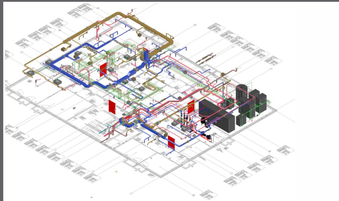
Isometrie TGA-Gesamtmodell Untergeschoss mit Technikzentrale Heizung und Sanitär
