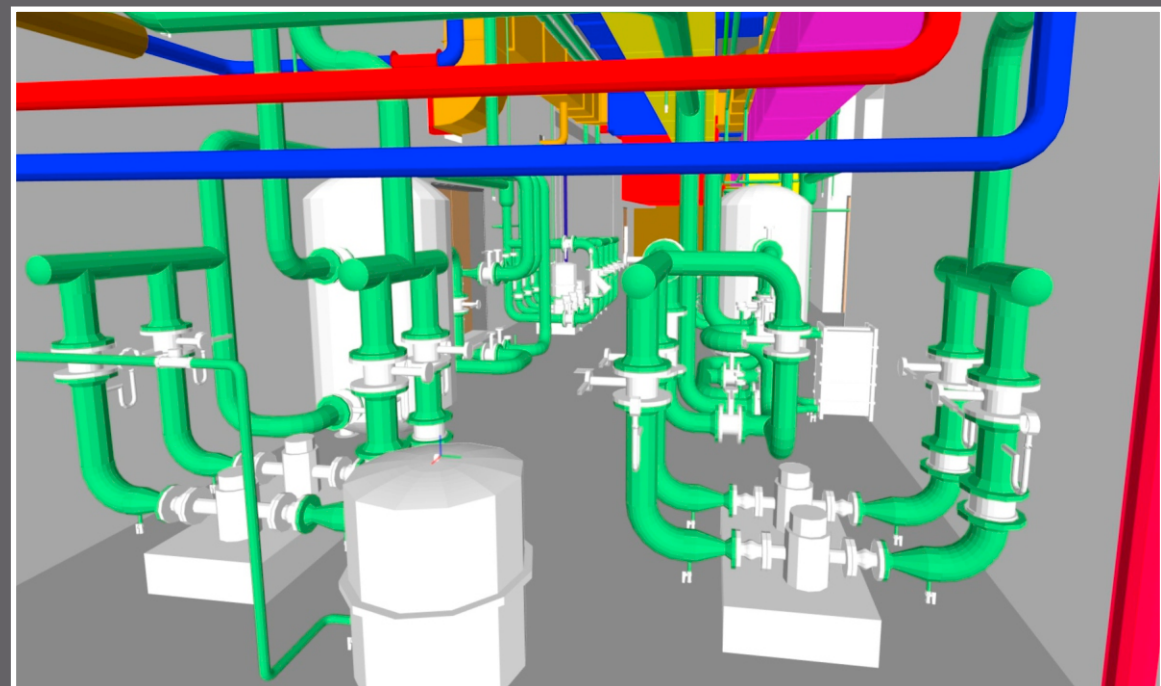
Kältezentrale im Untergeschoss Gesamtkälteleistung 335 kW
